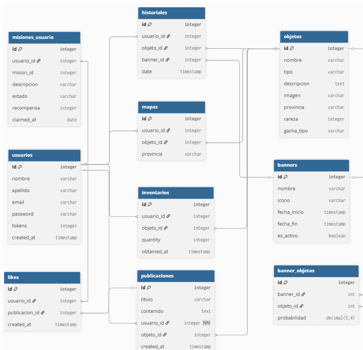
Figura 7: Diagrama de Base de Datos
