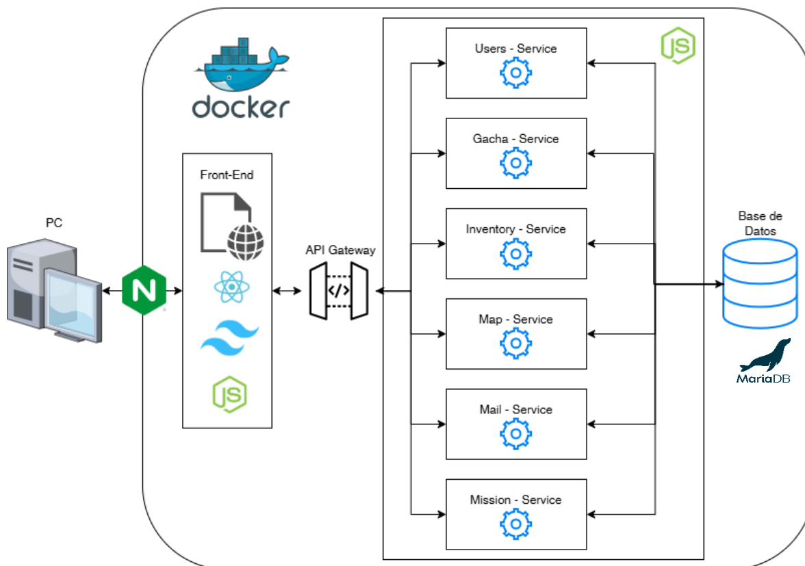
Figura 23: Arquitectura del Sistema
